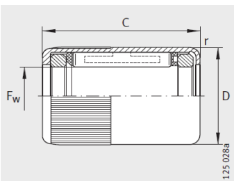
HFL0308-KF-R、 HFL0408-KF-R、 HFL0615-R、HFL0615-KF-R
