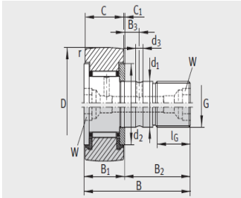
自 D = 22 mm KR (R = 500 mm) KR...PP (优化的 INA 轮廓)
