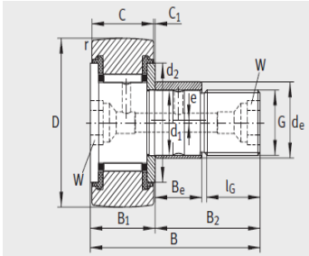
自 D = 22 mm KRE...PP (优化的 INA 轮廓形状)
