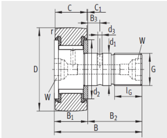
自 D = 22 mm KRV...PP (优化的 INA 轮廓形状)
