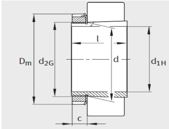
锥度为 1 : 12 (H240、H241 系列, 锥度为 1 : 30) 止动垫圈 MB
